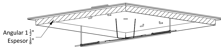
Isométrico 2 (visto desde parte inferior)
