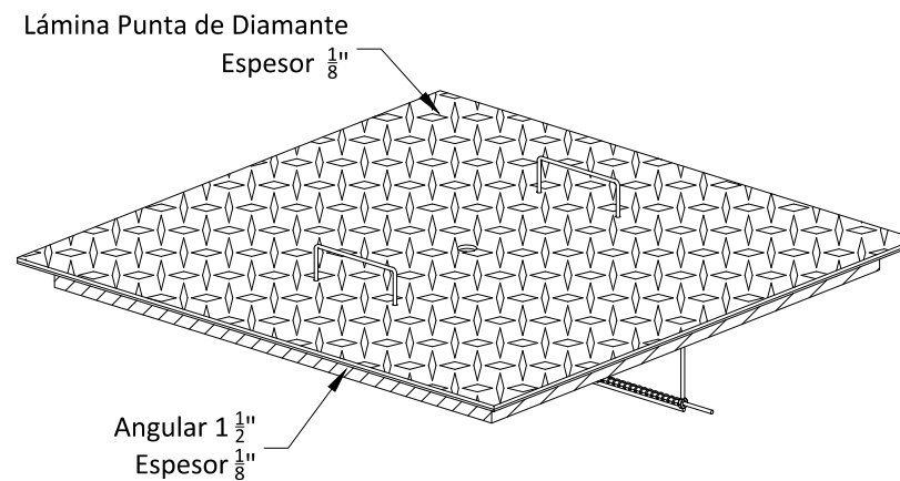
Isométrico 2 (visto desde parte superior)
