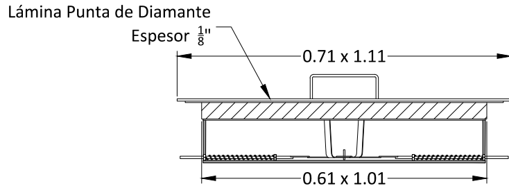
Elevación Frontal
