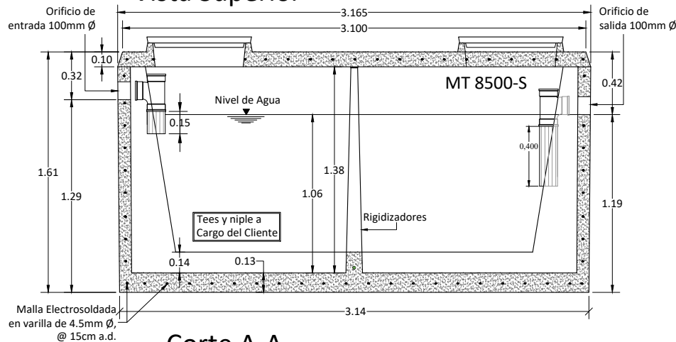
Corte A-A
