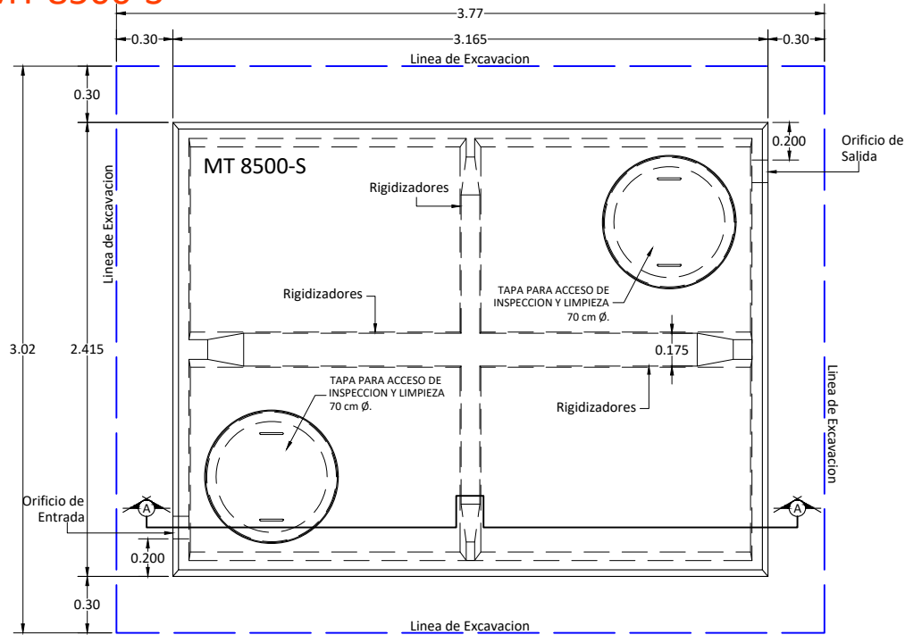
Vista Superior
