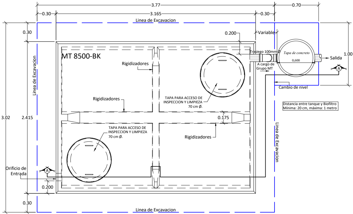
Vista Superior
