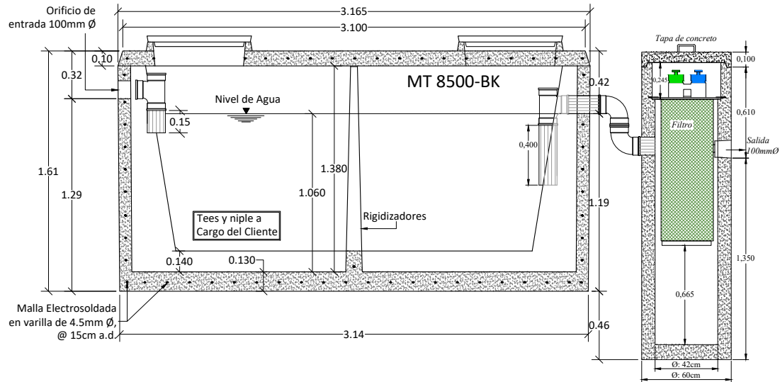
Corte A-A
