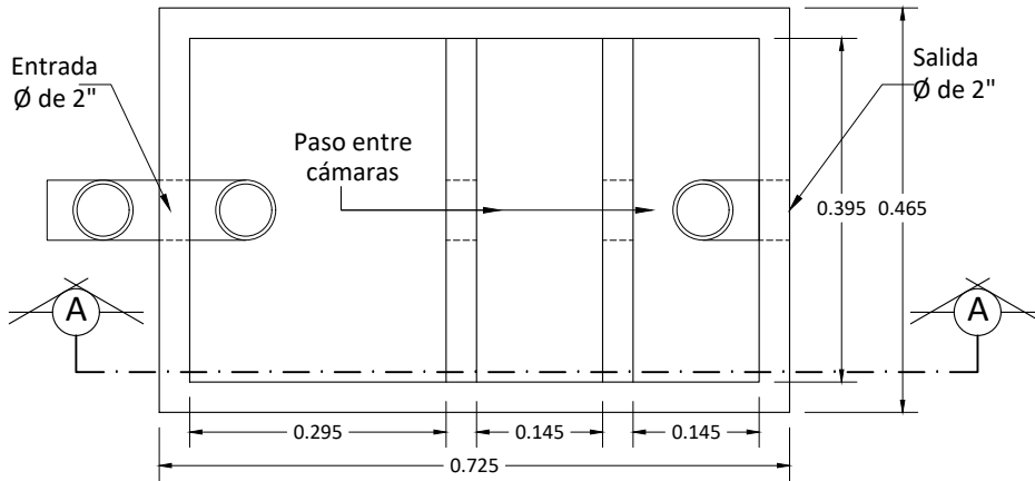
Vista Superior
