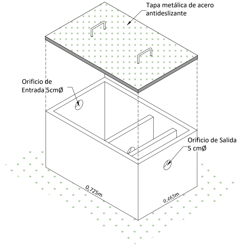
Isométrico
