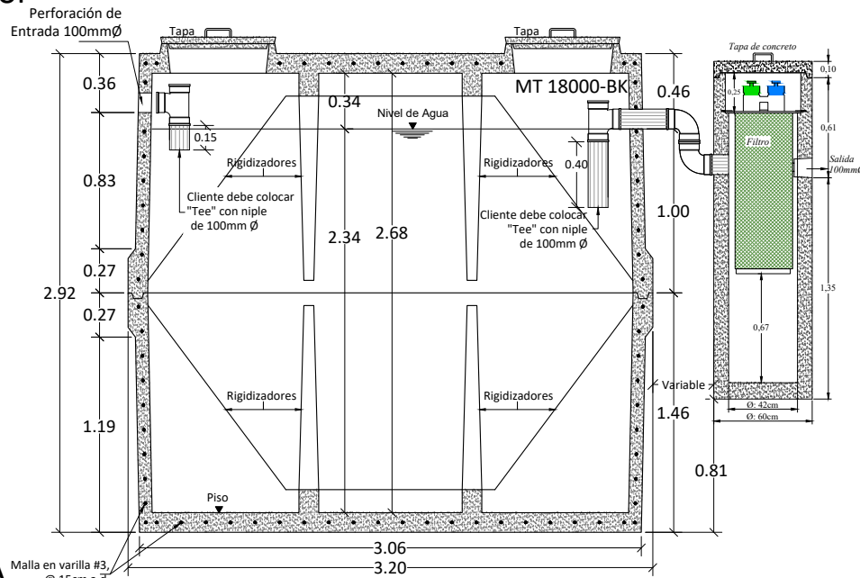
Corte A-A
