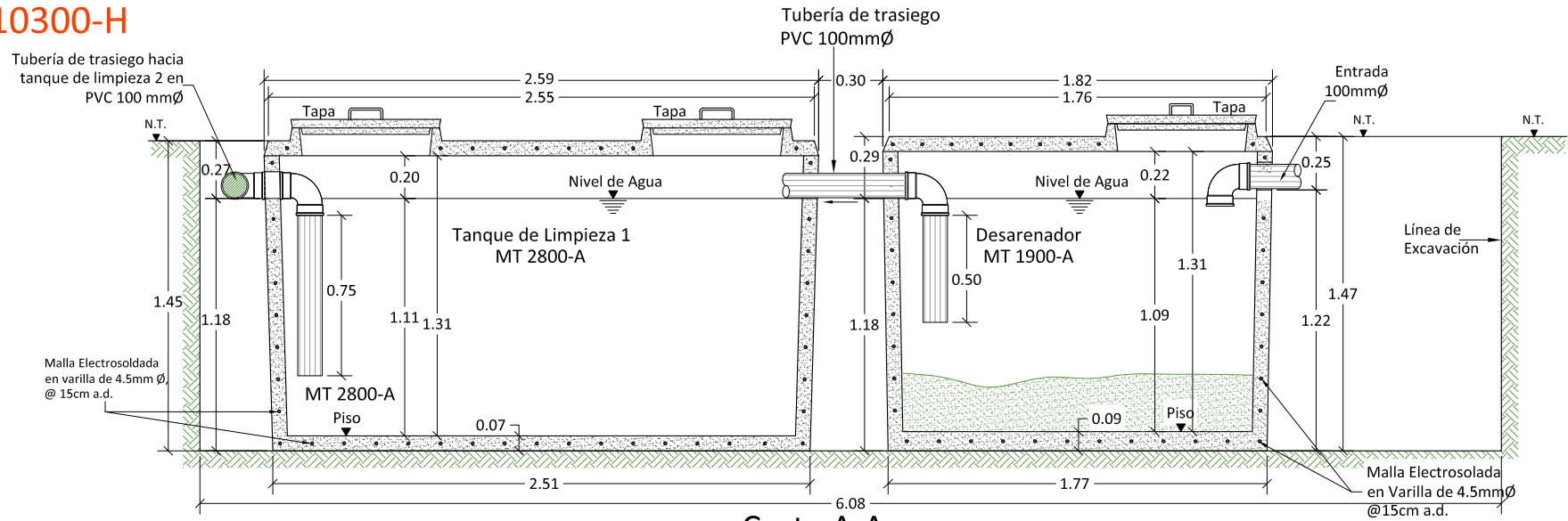
Corte A-A
