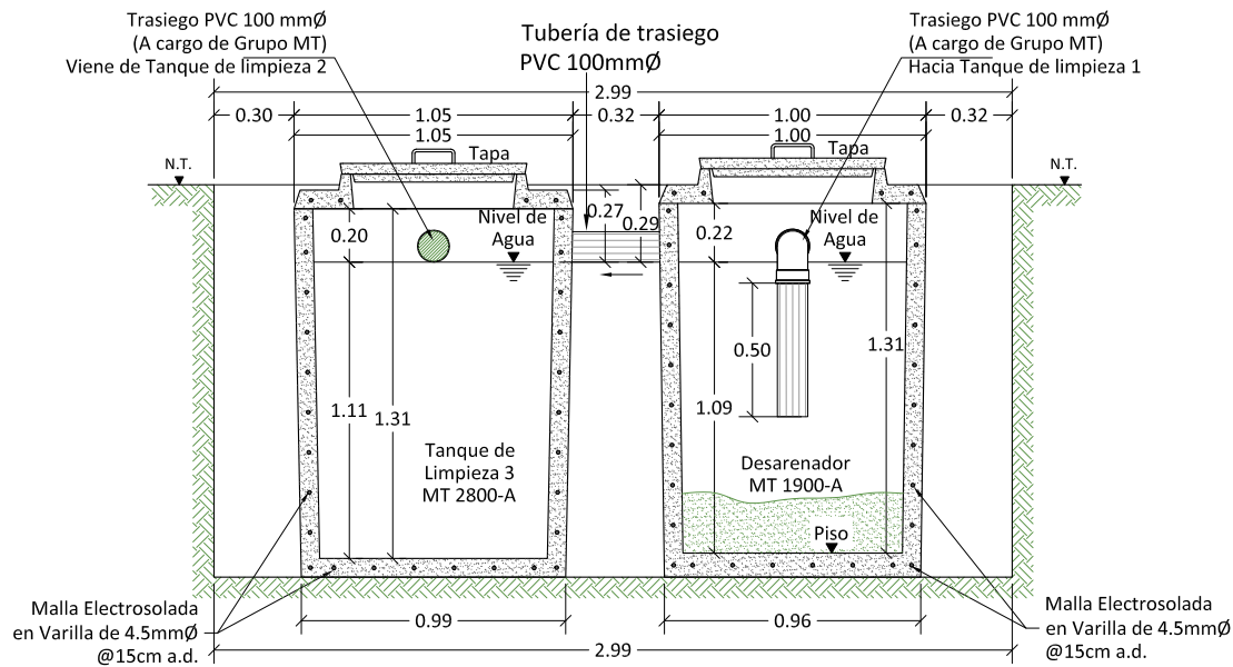
Corte B-B
