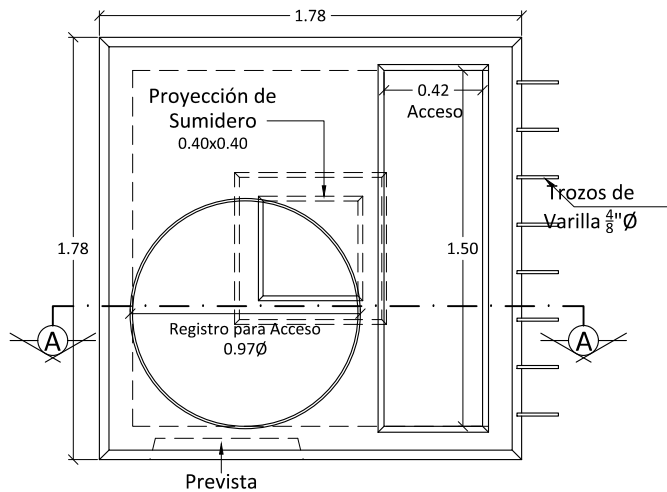
Vista Superior
