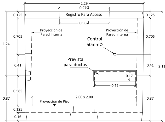
Elevación Lateral Derecha
