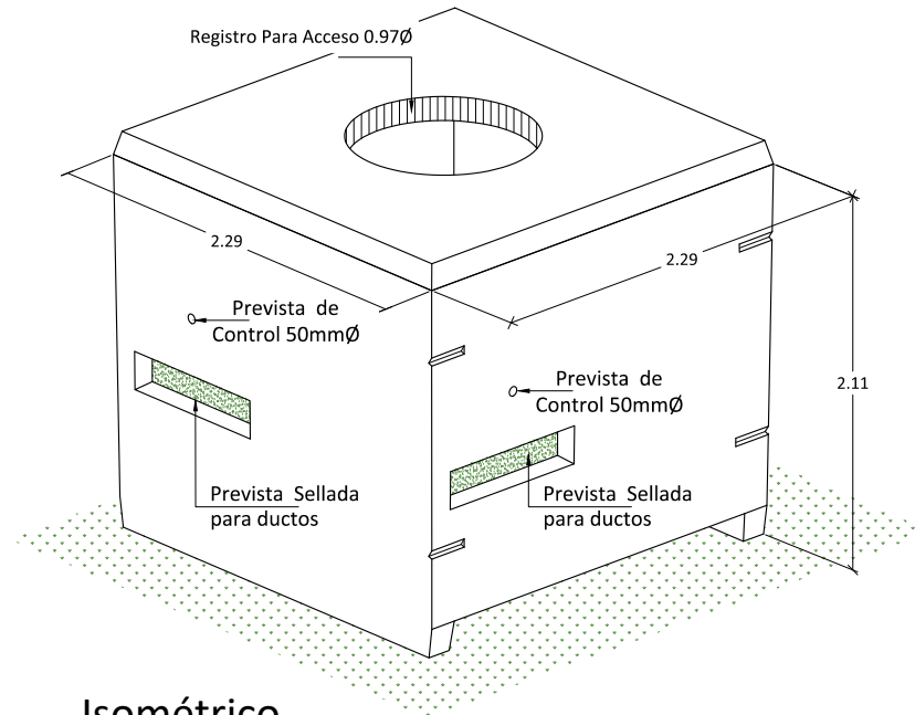
Isométrico
