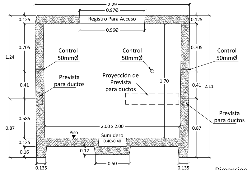
Corte A-A
