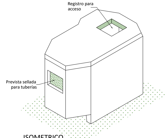
ISOMETRICO
