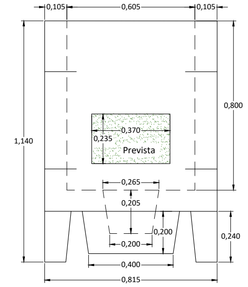
VISTA POSTERIOR
