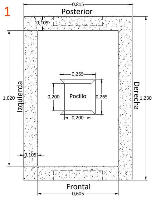
VISTA SUPERIOR
